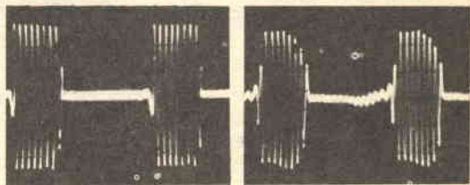
In alto: risposta con i controlli in varie posizioni. In basso a sinistra: distorsione alle frequenze basse. In basso a destra: fotografie di impulsi scattate alle frequenze di 100 Hz e 5.000 Hz.
