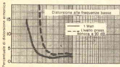
In alto: risposta con i controlli in varie posizioni. In basso a sinistra: distorsione alle frequenze basse. In basso a destra: fotografie di impulsi scattate alle frequenze di 100 Hz e 5.000 Hz.
