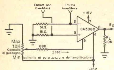
Fig. 4 - Amplificatore OTA a guadagno controllato.
